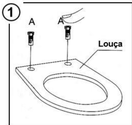
Insira nos orifícios da louça as buchas de expansão.
