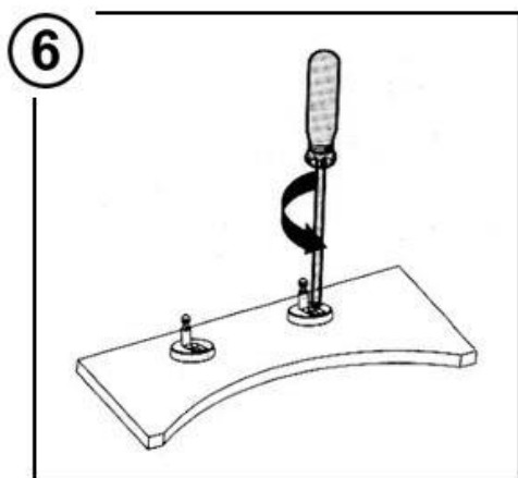
Aperte os parafusos da dobradiça
